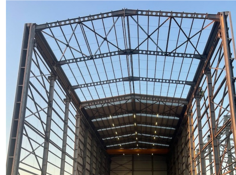
ÇELİK KONSTRUKSİYON
